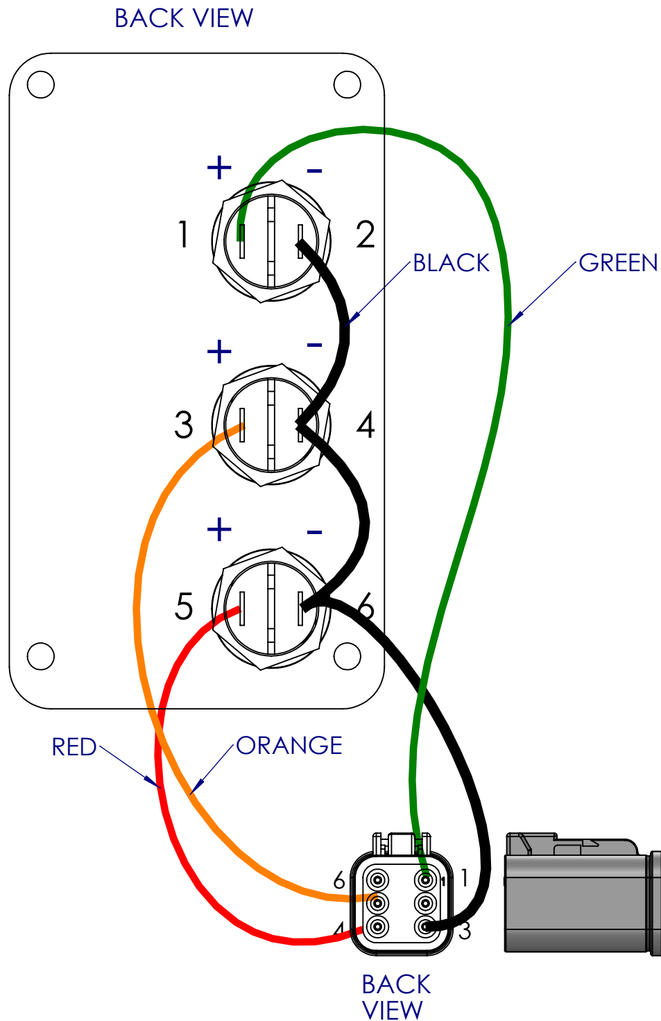
DEUTSCH DT06-6S
